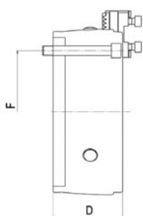
AUTOCENTRANTE DURO-T, A 3 GRIFFE: attacco a flangia, con griffe base e griffe reversibili
